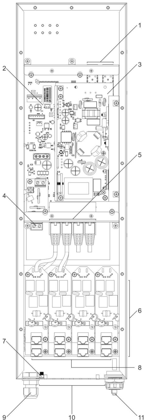
Рисунок 30 – Основные компоненты и разъемы MES3708P
